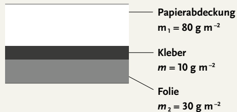
Abb. 8 Querschnitt einer selbstklebenden Folie
